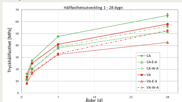
Figur 1. Hållfasthetsutveckling hos bruk (CA/VA=cementtyp, E/W=hydrofoberande medel, A=accelerator)
