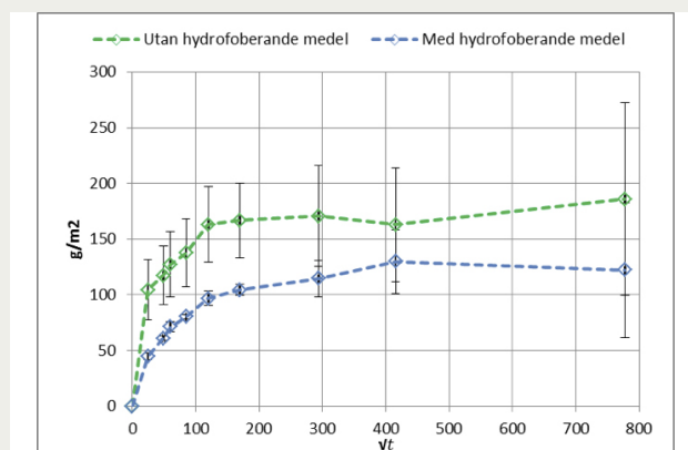
Figur 4. Absorptiviteten hos sprutbetongen.
